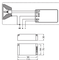
Scheda tecnica Osram PTi 1x70/220-240 S
