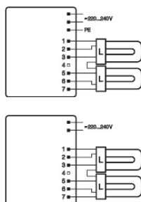
Scheda tecnica Osram QT-M 2X26-42/220-240 S
